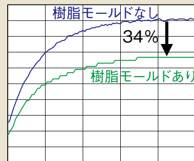
同一出力での温度上昇
